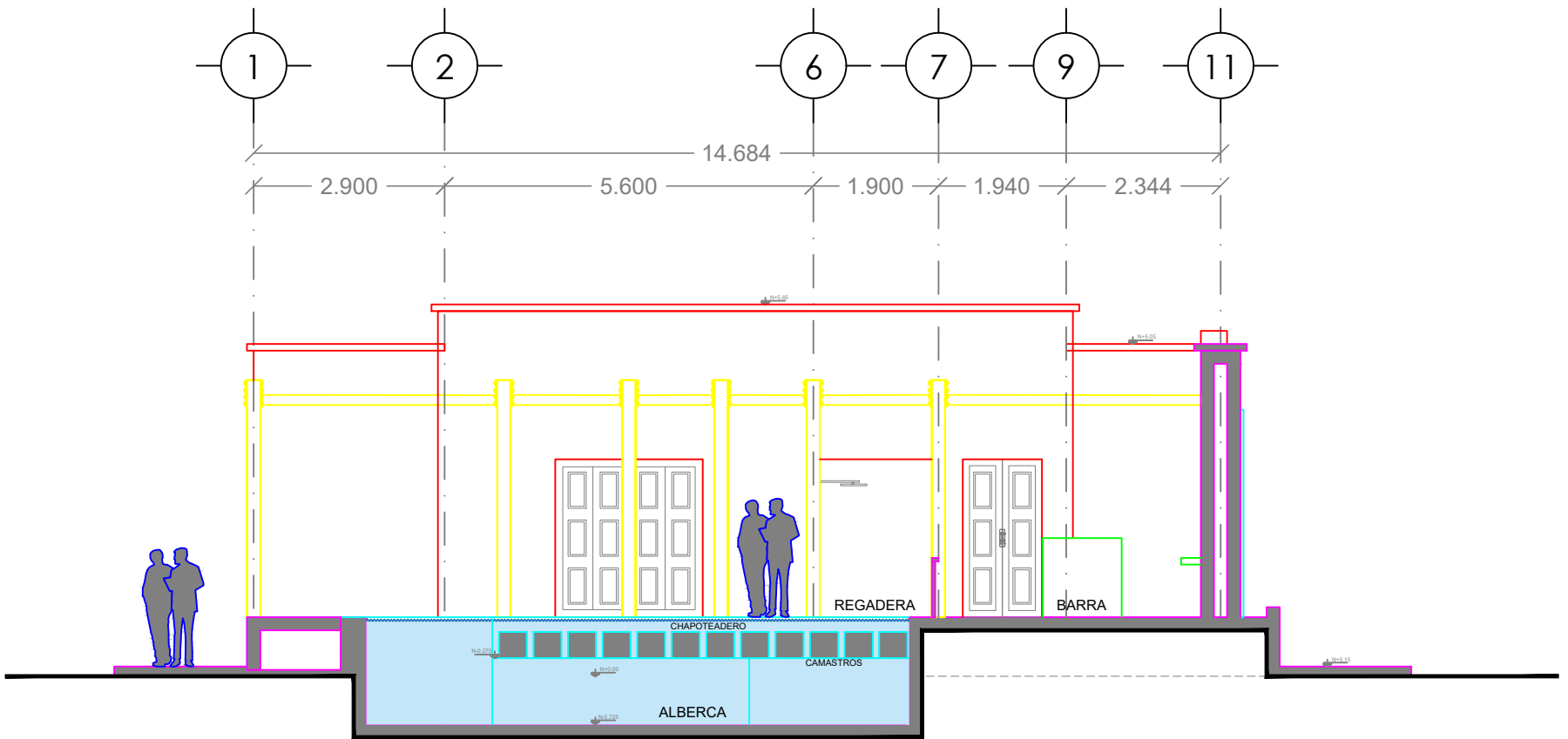
CORTE B-B'
